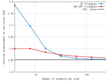
(b) TRI: displacement
