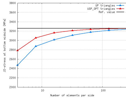
(d) TRI: J2-stress
